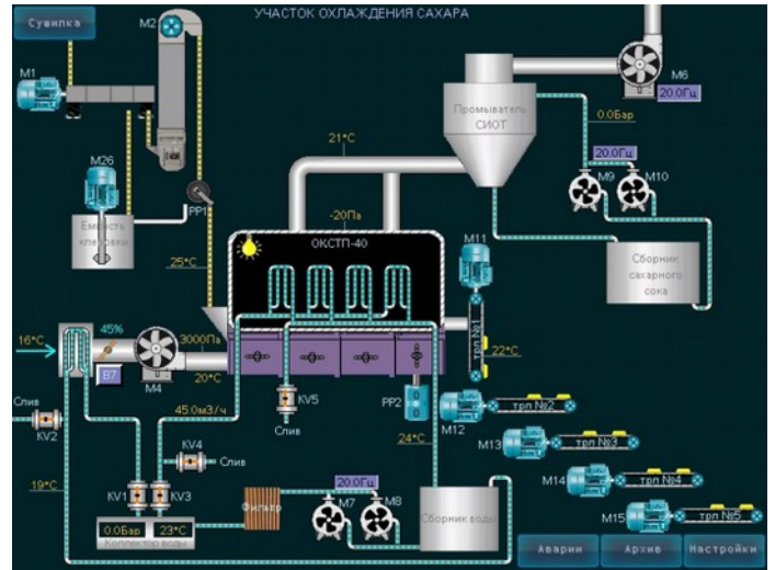
Панель управления. Узел охладителя
