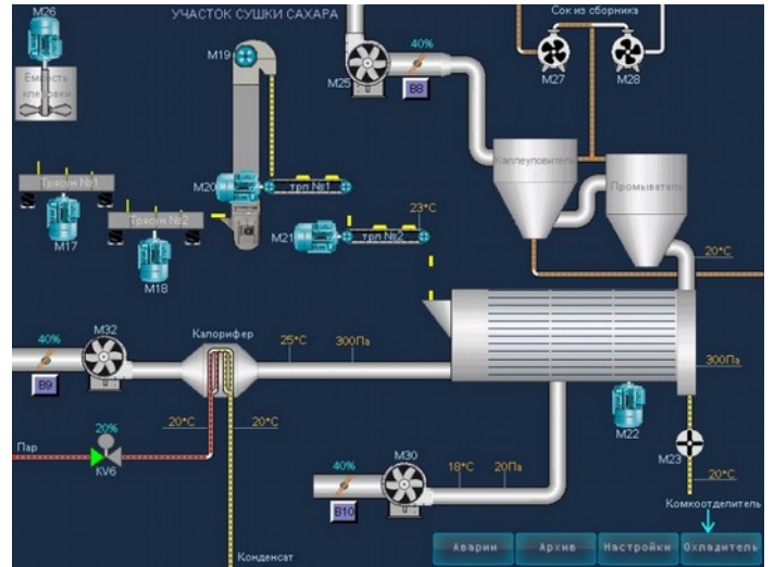
Панель управления. Узел суши
